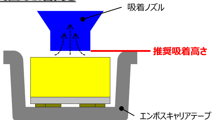
図5. 推奨吸着高さ
