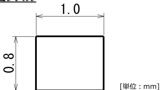
図3. 参考吸着ノズル外形
