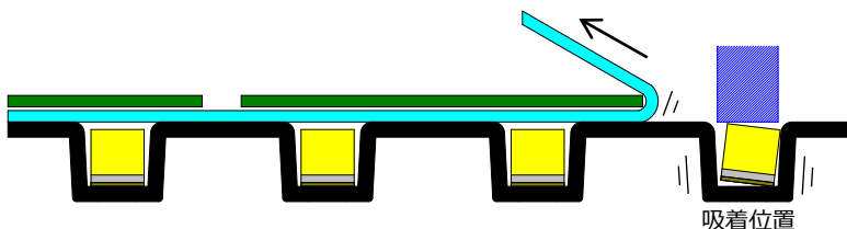
図4. カバーテープ剥離位置について
