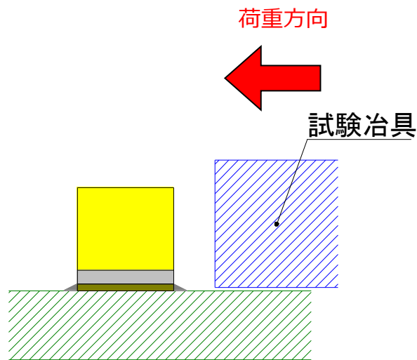
図10. 試験方法
