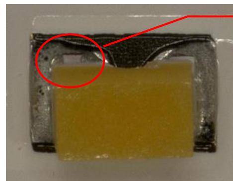
図11. 試験後外観
