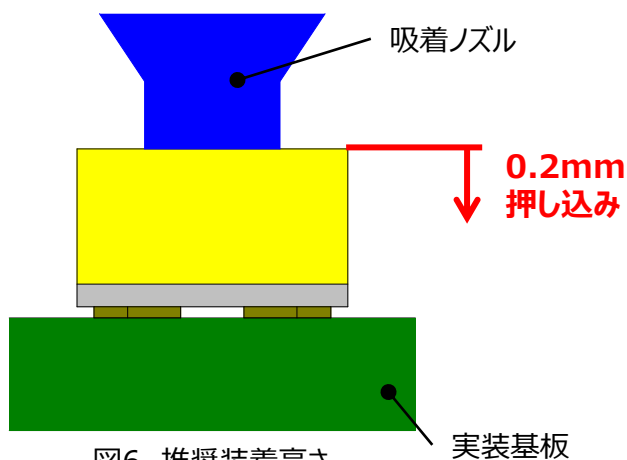
図6. 推奨装着高さ
